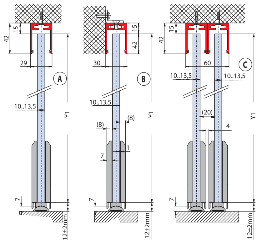
Схема стеклянных раздвижных дверей к стене и потолку
